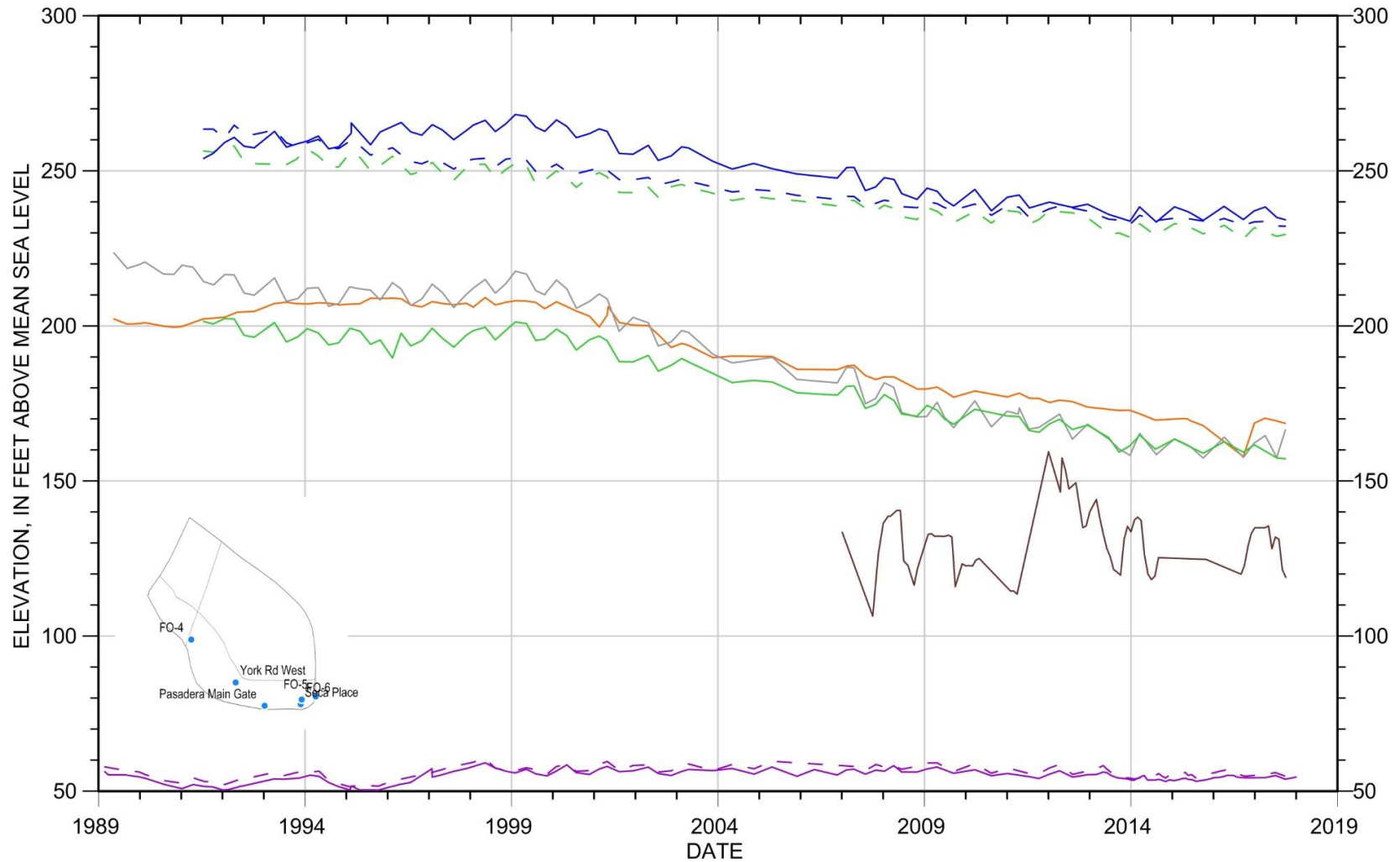
Figure 9. Laguna Seca Subarea Hydrographs
